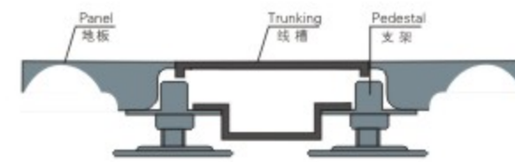
线槽地板安装示意图
